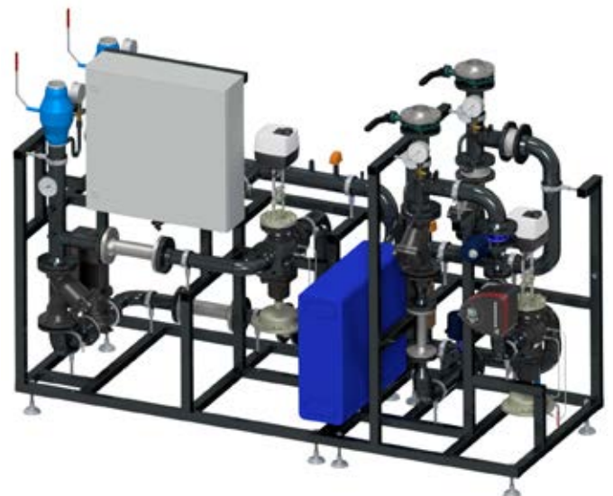
450 kW aqoFrame bidirektional zur Möglichkeit der Rückspeisung von Wärme ins Netz
