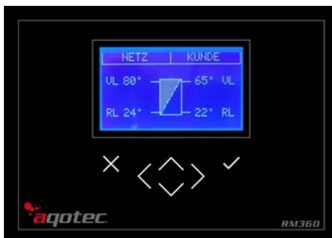
Bedienteil RM360 für Fronteinbau (Normausschnitt)
