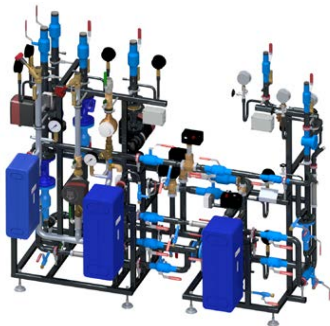
306 kW aqoFrame mit Trinkwasser Vor- und Nachwärmer zur Absenkung der Rücklauftemperatur und zwei gemischten Heizkreisen
