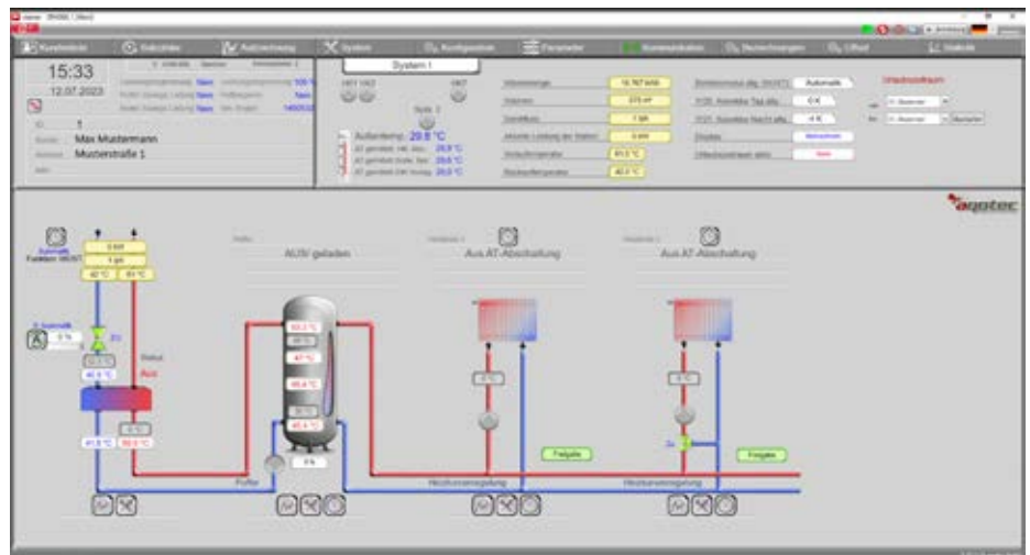
Die aqo360° Kundenanlagenvisualisierung ermöglicht es den Anlagenstatus zu prüfen, Parameter zu verändern und historische Daten auszuwerten.
