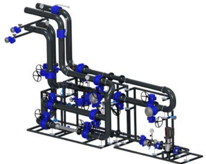
Beimischstation zur Absenkung der Vorlauftemperatur in einem speziellen Fernwärmenetz
